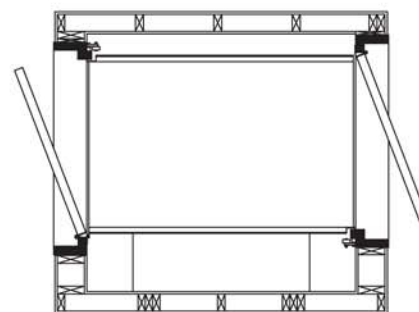
Vue de dessus en coupe (élévateur et puits)
