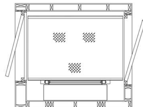
Vue de dessus en coupe
