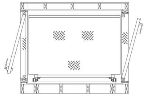
Vue de dessus en coupe (Élévateur et puits)
